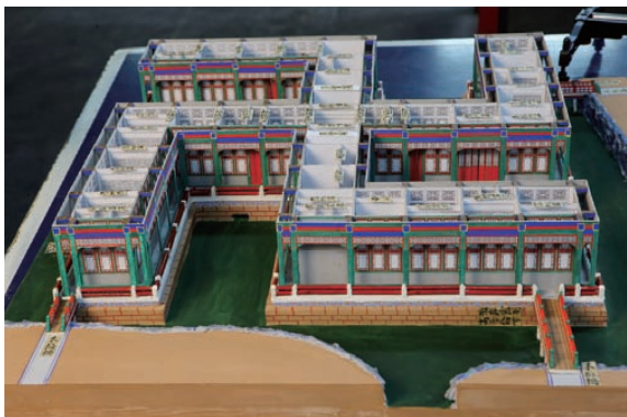
㉔ 建物の配置や室内意匠の設計に用いる紙模型
